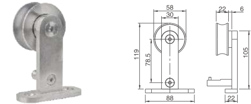
TR04-W2 For Glass Door
